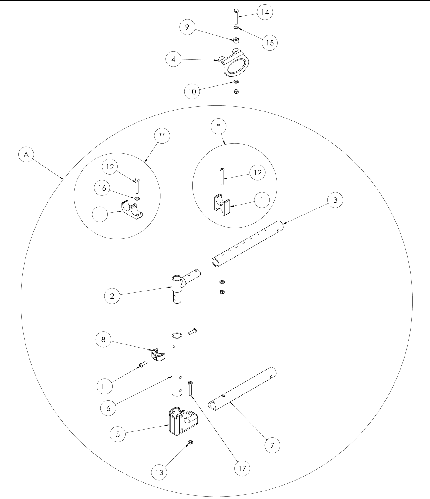
1 ASSEMBLAGE GAUCHE ILLUSTRÉ
