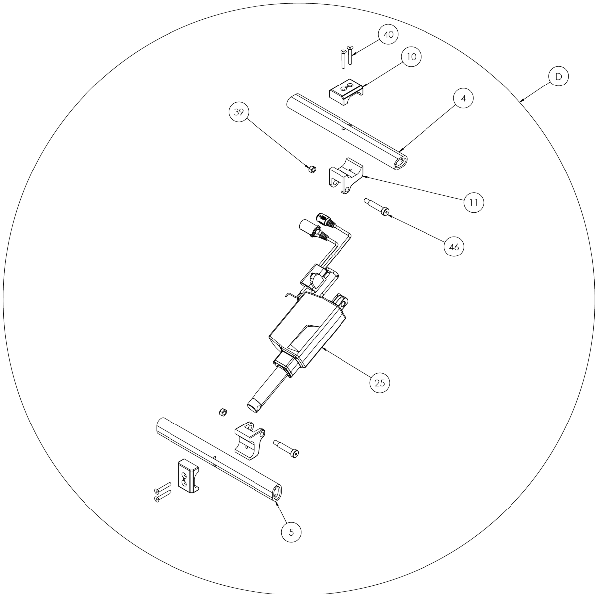
DÉTAIL / DETAIL D ÉCHELLE / SCALE 1:3
