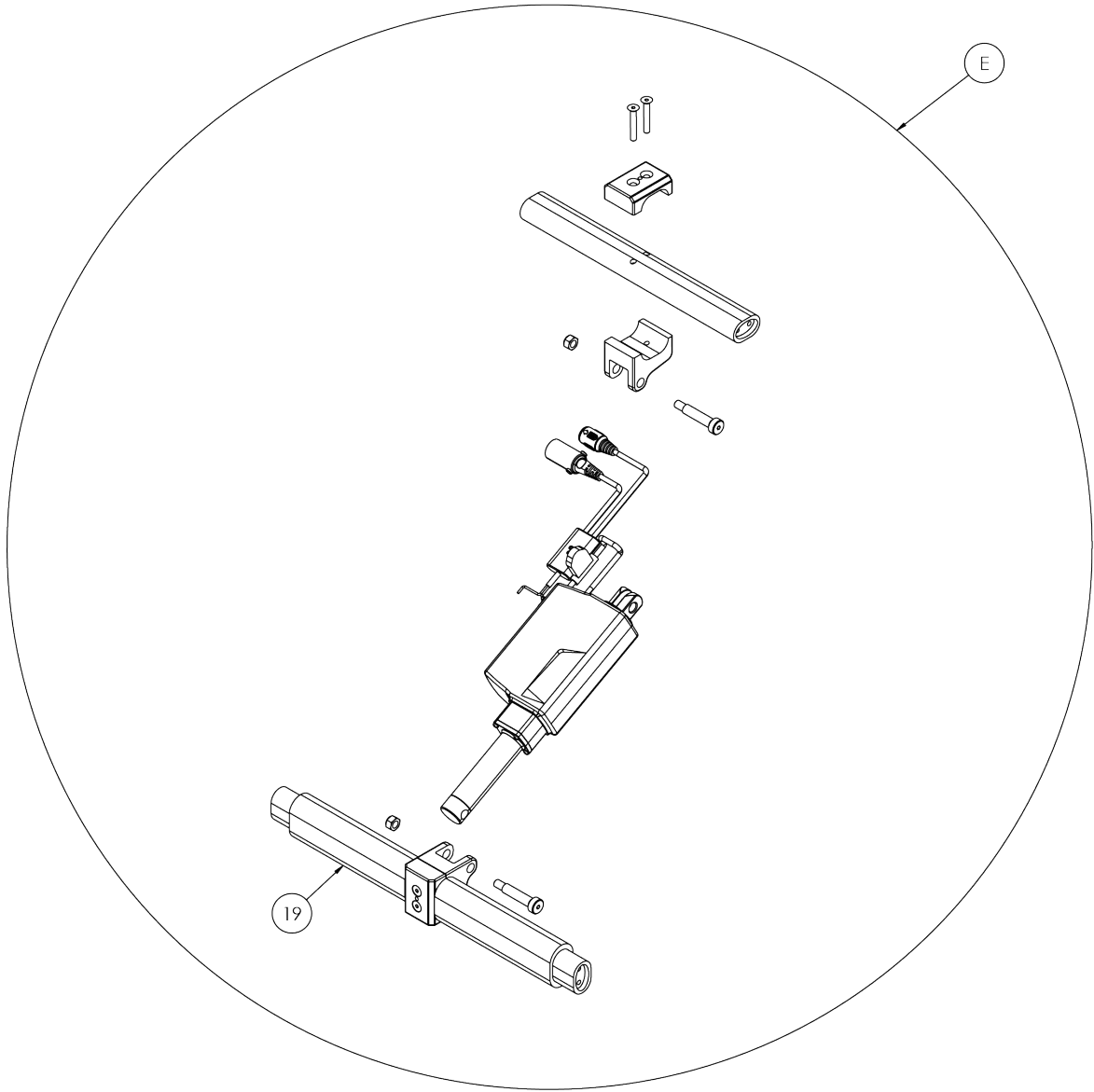
DÉTAIL / DETAIL E ÉCHELLE / SCALE 1:3
